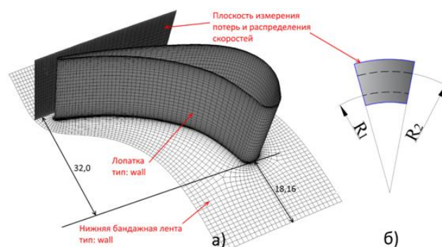
Figure 11 Внешний вид расчетной схемы
