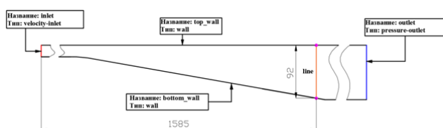
Figure 3 Расчетная схема исследуемого канала
