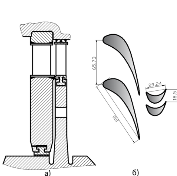
Figure 7 Ступень паровой турбины (а) и характеристики сопловой и рабочей решеток на среднем сечении (б)
