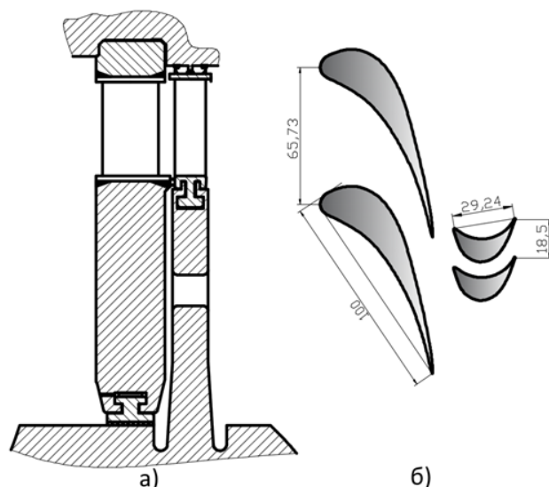
Figure 7 Ступень паровой турбины (а) и характеристики сопловой и рабочей решеток на среднем сечении (б)
