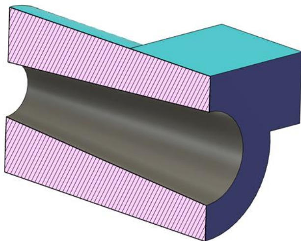
Figure 6 Внутренняя часть циклона
