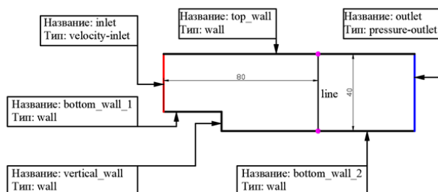
Figure 9 Геометрия расчетной области
