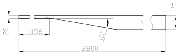
Figure 2 Геометрические характеристики исследуемого диффузора
