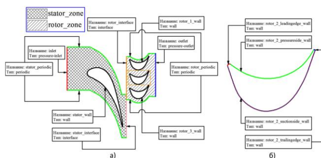
Figure 8 Расчетная схема
