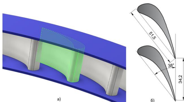
Figure 10 Внешний вид сопловой решетки (а) и геометрические характеристики межлопаточного канала на среднем диаметре (б)
