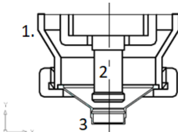
Figure 1 Катодный узел
