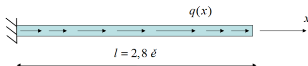
Figure 4 В каких сечениях следует поставить три тензодатчика, чтобы определить наиболее достоверно среднюю деформацию стержня?
