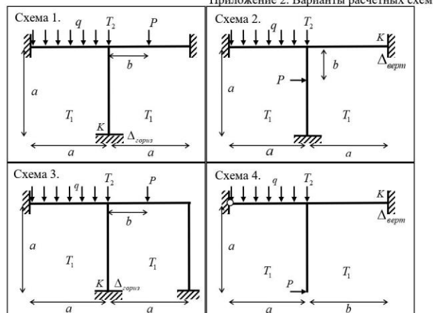
Приложение 2. Варианты расчетных схем
