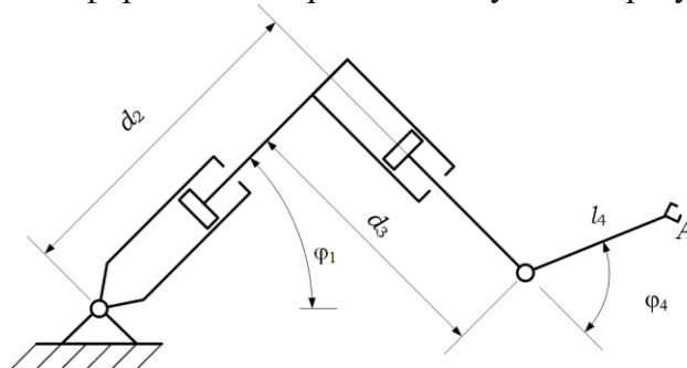
Figure 7 Схема манипулятора
