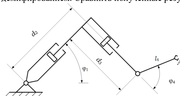
Figure 8 Схема манипулятора
