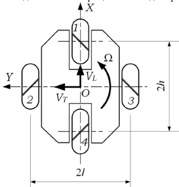
Figure 1 Схема омни-платформы
